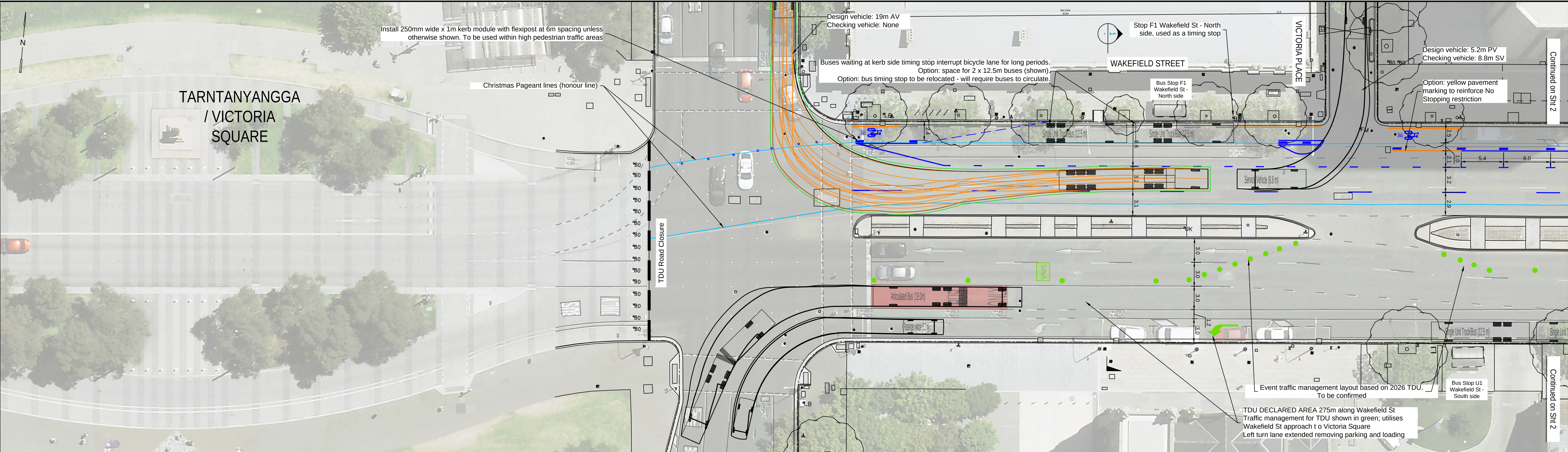
Plan 1:250
